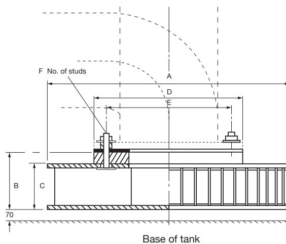
Suction Lifts B.S. 4504 Table PN 16. Dimensions mm:
